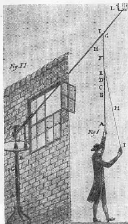
Опыт А. Вольты по измерению электризации воздуха.
