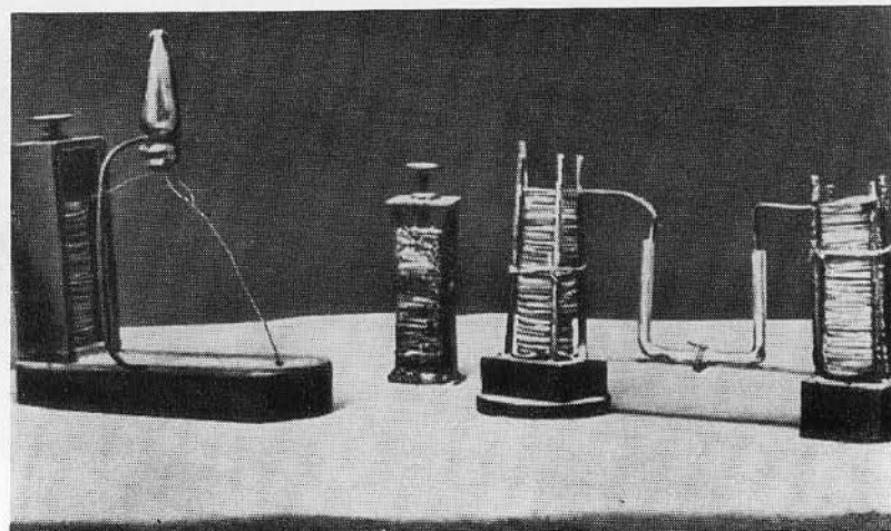
Вольтовы столбы различного назначения.
