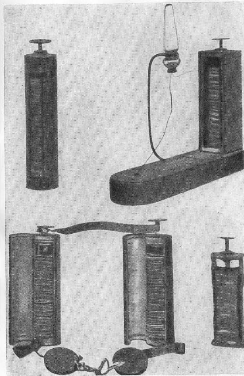
Вольтовы столбы усовершенствованной конструкции.
