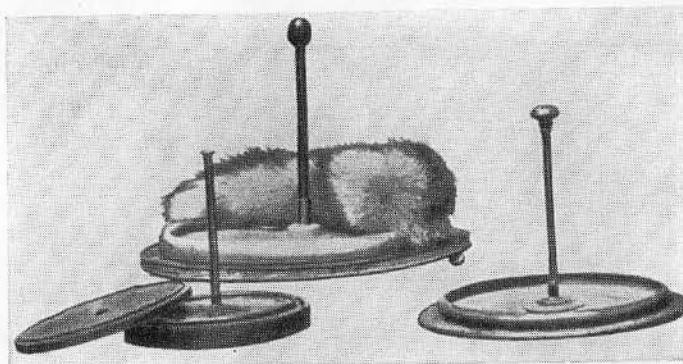
Электрофоры, построенные А. Вольтой в 1775—1780 годах.
