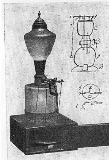
Эвдиометры разного назначения, сконструированные А. Вольтой.
