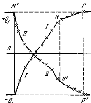
Рис. 2. Кривые зависимости количества электричества на пластине от времени между пропусканием излучения и переменной направления поля
