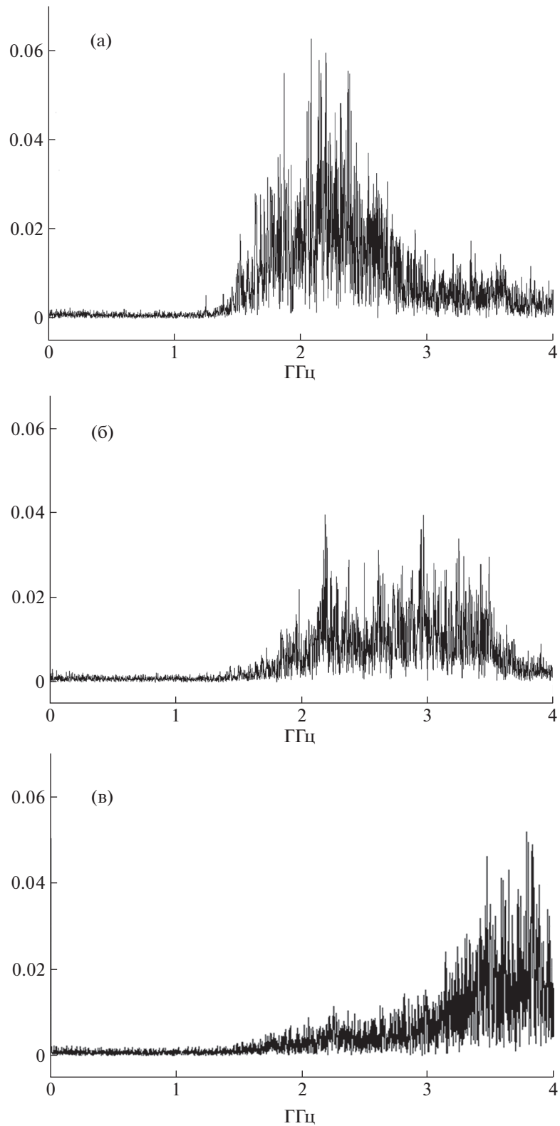
Рис. 2. Спектры излучения плазменного релятивистского СВЧ-усилителя шумов РЭП для разных значений плотности плазмы. Плотность плазмы увеличивается от верхнего графика к нижнему. Энергия СВЧ-импульсов 5–10 Дж.
