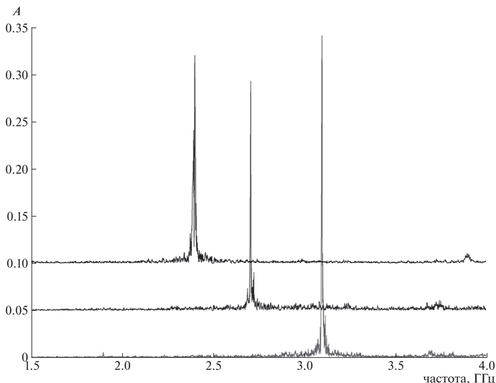
Рис. 1. Спектры плазменного релятивистского СВЧ-усилителя для частот входного сигнала 2.4, 2.7 и 3.1 ГГц. Мощность входного сигнала около 50 кВт, максимальная мощность излучения в импульсе 100–150 МВт. Спектры сигналов на частотах 2.7 и 2.4 ГГц смещены вверх на 0.05 отн. ед.
