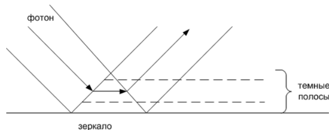
Рис. 1. Отражение фазовой волны де Бройля от плоского зеркала
